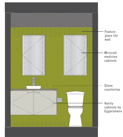
ENSUITE ELEVATION A
