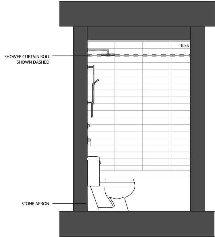
ELEVATION B
