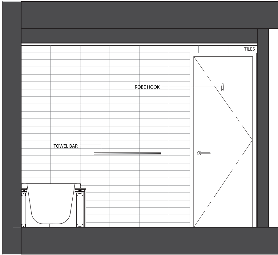
ELEVATION A
