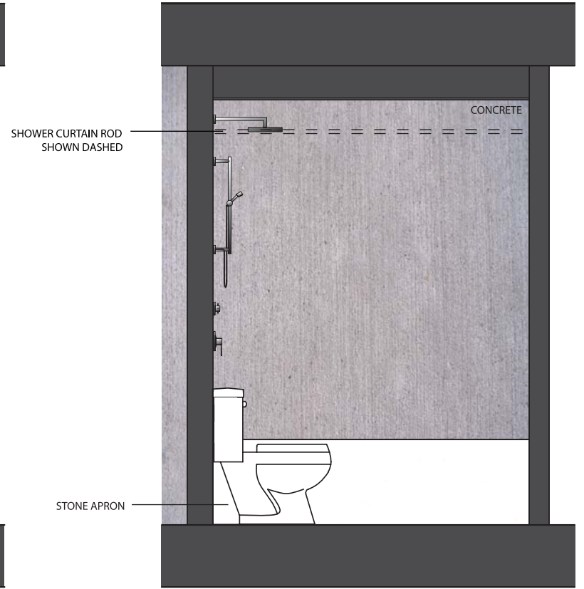
ELEVATION B
