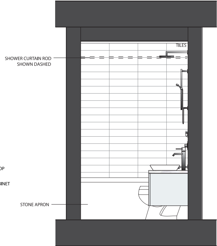
ELEVATION B
