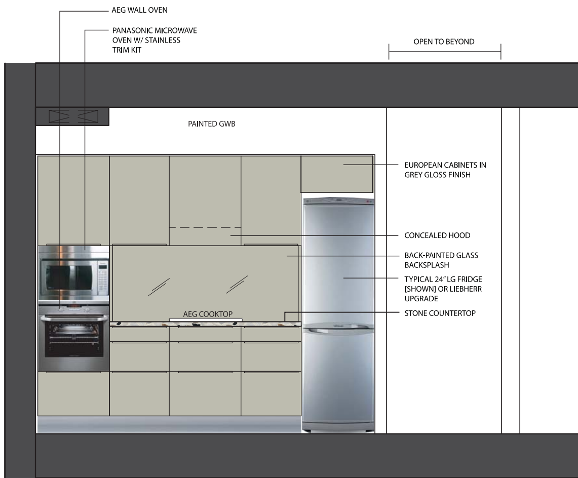
ELEVATION A
