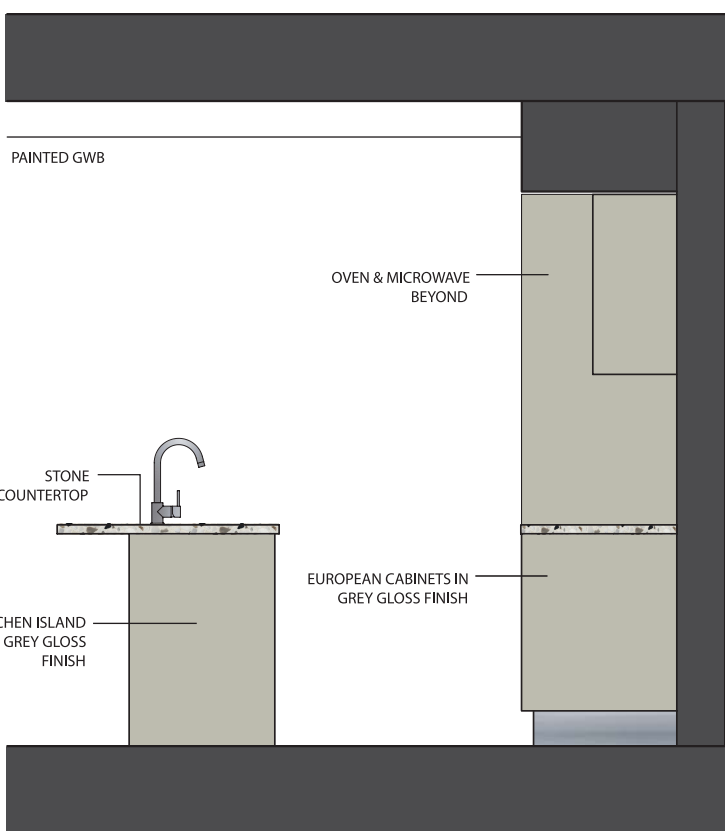
ELEVATION B
