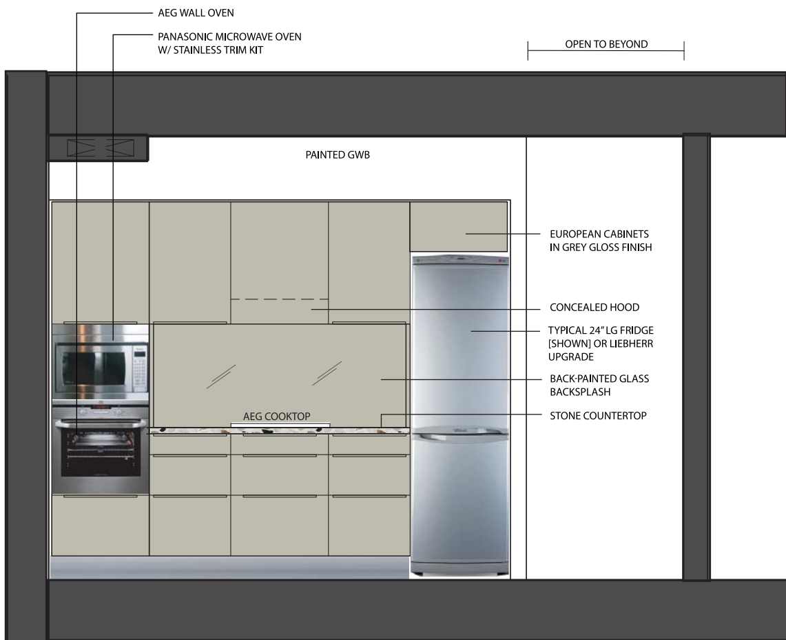
ELEVATION A
