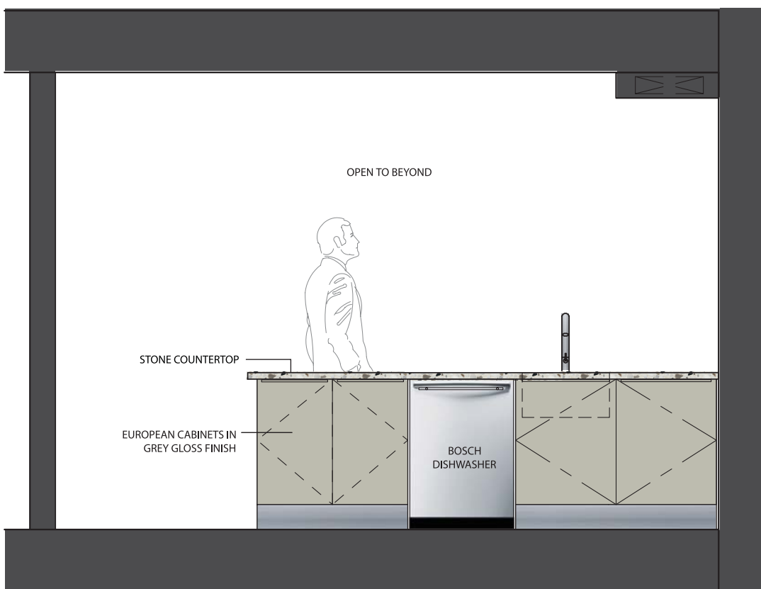
ELEVATION B
