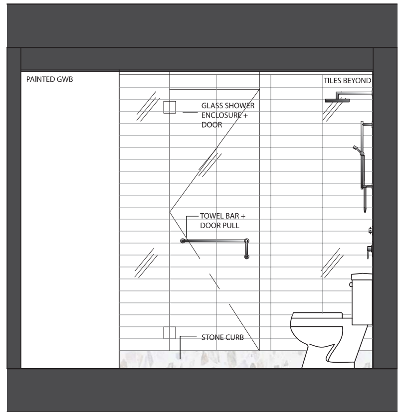
ELEVATION B
