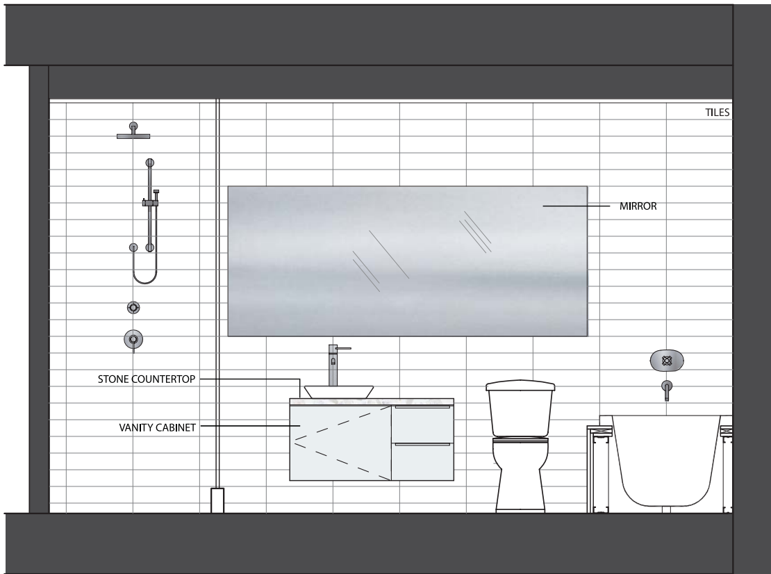
ELEVATION A
