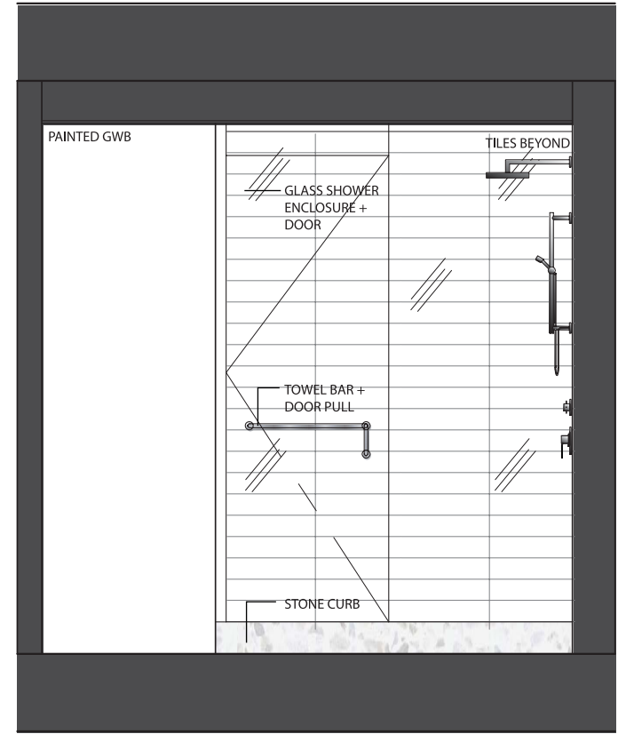
ELEVATION B
